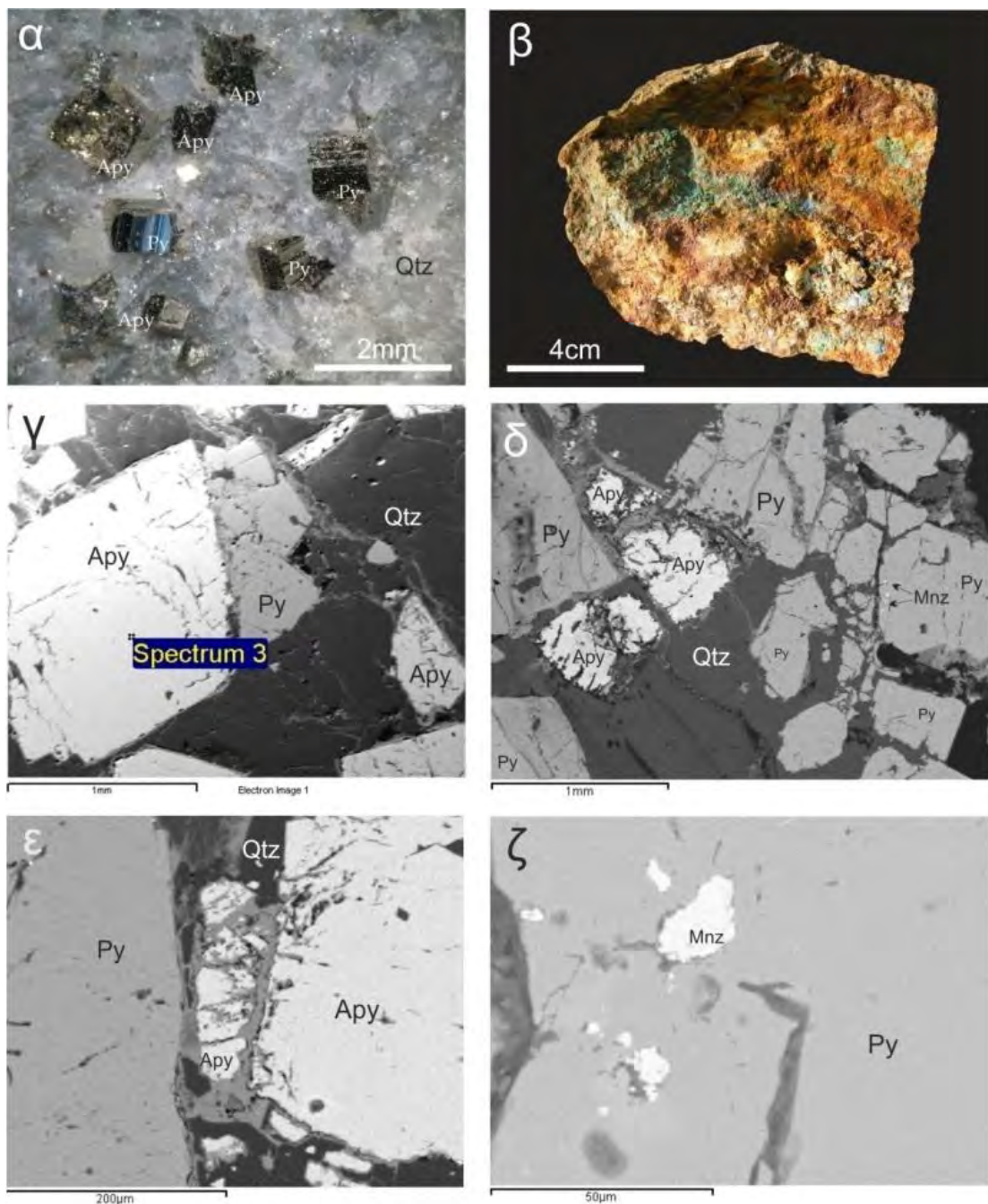
Εικόνα 8.6.10.1 α) Κρύσταλλοι αρσеноπυρίτη (Apy) και σιδηροπυρίτη (Py) σε χαλαζία (Qtz) από την πρωτογενή μεταλλοφορία στις Ασημότρυνες. Εικόνα από στερεοσκόπιο. β) Οξειδωμένη μεταλλοφορία με γκαιίτη, μαλαχίτη και αζουρίτη. γ) Αρσеноπυρίτης (Apy) σε σύμφυση με σιδηροπυρίτη (Py). SEM, back-scattering image. δ) Αρσеноπυρίτης (Apy) και σιδηροπυρίτης (Py) με κατακλαστική υφή σε χαλαζία (Qtz). Διακρίνονται κόκκοι μοναζίτη (Mnz) μέσα στο σιδηροπυρίτη. SEM, back-scattering image. ε) Κρύσταλλοι σιδηροπυρίτη (Py) και αρσеноπυρίτη (Apy). Στο αριστερό του άκρο ο κρύσταλλος του αρσеноπυρίτη οξειδώνεται περιφερειακά και στις κατακλάσεις σε οξείδιο του Fe-As. SEM back-scattering image. ζ) Έγκλεισμα μοναζίτη (Mnz) σε σιδηροπυρίτη (Py). SEM, back-scattering image.
