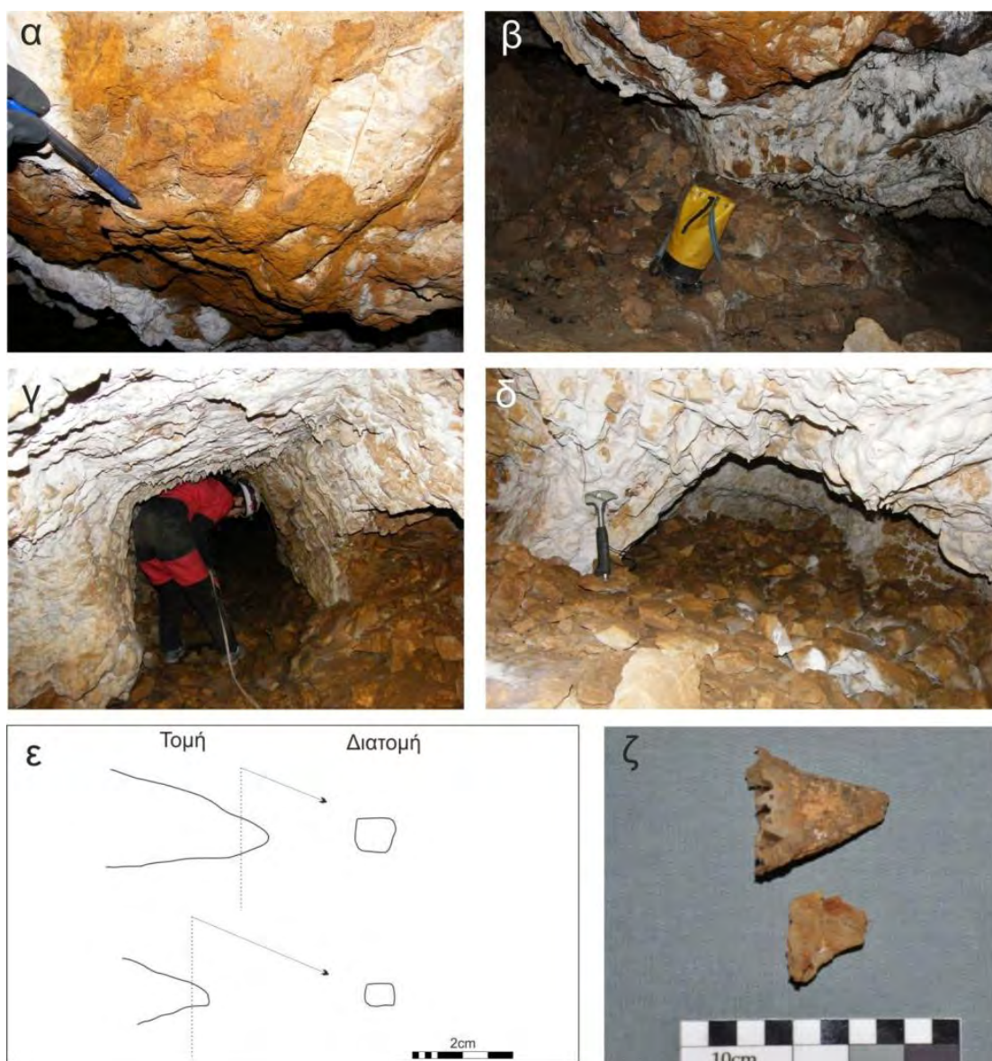
Εικόνα 8.1.3.3 α) Ίχνη της εκμετάλλευσης στα τοιχώματα της στοάς Κοκκινόχωμα-1. β) Τοίχιο υποστήριξης δομημένο από στείρο υλικό της εξόρυξης. γ) Αποψη της στοάς Κοκκινόχωμα-1. δ) Πλήρωση τμήματος της στοάς με στείρο εξορυγμένο υλικό. ε) Τομές και διατομές από τα ίχνη του μεταλλευτικού σφυριού. ζ) Θετικά εκμαγεία εργαλείων εξόρυξης από το εσωτερικό της στοάς.
