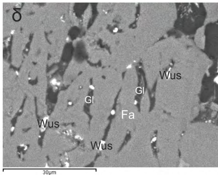
Εικόνα 9.3.2.2 Φωτογραφίες σε μικροσκόπιο από σκωρίες στη μεταλλουργική θέση Παλαιοχωρίου α) Βουσιτίτης (Wus) σε φαυαλίτη (Fa). Οι βαθύχρωμες φάσεις είναι η υαλώδης μάζα (Gl), ενώ διακρίνονται οι σπές της σκωρίας. Μεταλλογραφικό μικροσκόπιο, N//. β) Η φωτογραφία 9.3.5α με πολωτικό μικροσκόπιο. Διακρίνονται οι επιμήκεις κρύσταλλοι του φαυαλίτη. N//. γ) Φαυαλίτης (Fa) μέσα σε υαλώδη μάζα (Gl). Με λευκό χρώμα διακρίνεται ο βουσιτίτης (Wus). SEM Back scattering image. δ) Επιμήκεις κρύσταλλοι φαυαλίτη (Fa) μέσα σε υαλώδη μάζα (Gl). Με λευκό χρώμα διακρίνεται ο βουσιτίτης (Wus). SEM Back scattering image.
