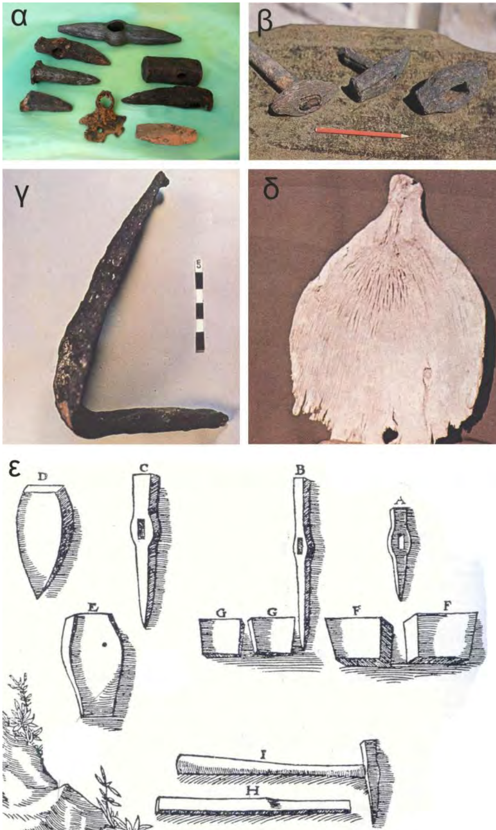
Εικόνα 3.7.3.2 α) Ρωμαϊκά μεταλλευτικά σφυριά, καλέμια και τσάπα (barryyeoman.com/2010/09/the-mines-that-built-empires/ φωτογρ. Aquilino Delgado). β) Σφυριά από το αρχαίο Λαύριο (Κονοφάγος, 1980). γ) Τσάπα από το αρχαίο Λαύριο (Κονοφάγος, 1980). δ) Φτυάρι από το αρχαίο Λαύριο (Κονοφάγος, 1980). ε) Α-Δ: μεταλλευτικά σφυριά, Ε: σφήνα, Γ:σιδερένια τεμάχη, F: σιδερένια πλακέτα, Ι-Η: στειλιάρια (Agricola, Hoover and Hoover, 1950).
