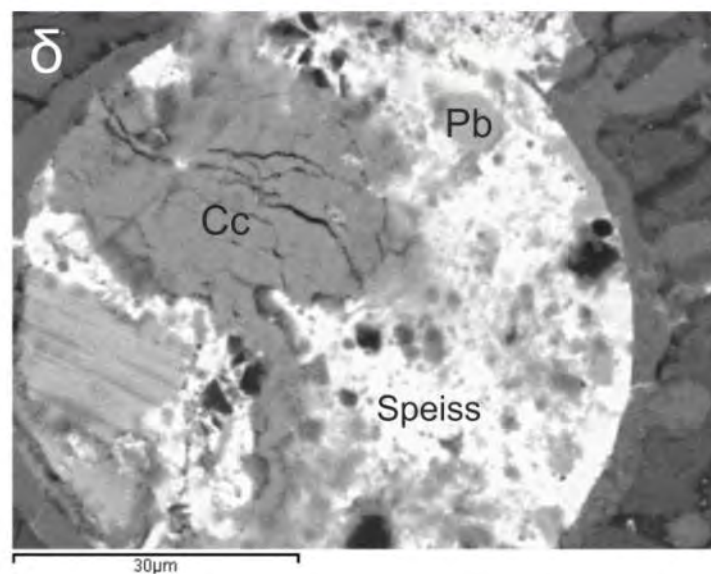
Εικόνα 9.1.2.1 Φωτογραφίες από μεταλλουργικές σκωρίες στο λόφο Σίνα. α) Κοκκίο αποτελούμενο από SPEISS μέσα στη μάζα της μεταλλουργικής σκωρίας. Μεταλλογραφικό μικροσκόπιο //N. β) Δενδριτικός βουστίτης (Wus) με κιρσταϊνίτη (Kir) σε ναλώδη μάζα (Gl). Διακρίνονται τα σφαιρίδια από speiss και μολύβδο (Pb) (λευκοκίτρινο χρώμα). Μεταλλογραφικό μικροσκόπιο //N. γ) Δενδριτικός βουστίτης (Wus), με κιρσταϊνίτη (Kir) μέσα σε ναλώδη μάζα (Gl). Διακρίνονται σφαιρικά κοκκία Speiss με περιεκτικότητες σε Cu από 1 έως 11%. SEM, back scattering image. δ) Κοκκίο Pb και Speiss με περιεκτικότητα σε Cu έως και 18%. Διακρίνεται ο χαλκοσύνης (Cc) με κατάκλαστική υφή. SEM, back scattering image.
