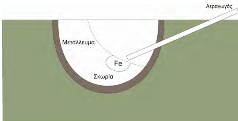
Εικόνα 3.8.6.1 Αναπαράσταση της φωλεόσχημης καμίνου. Τροποποιημένο από Tylecote (1987).
