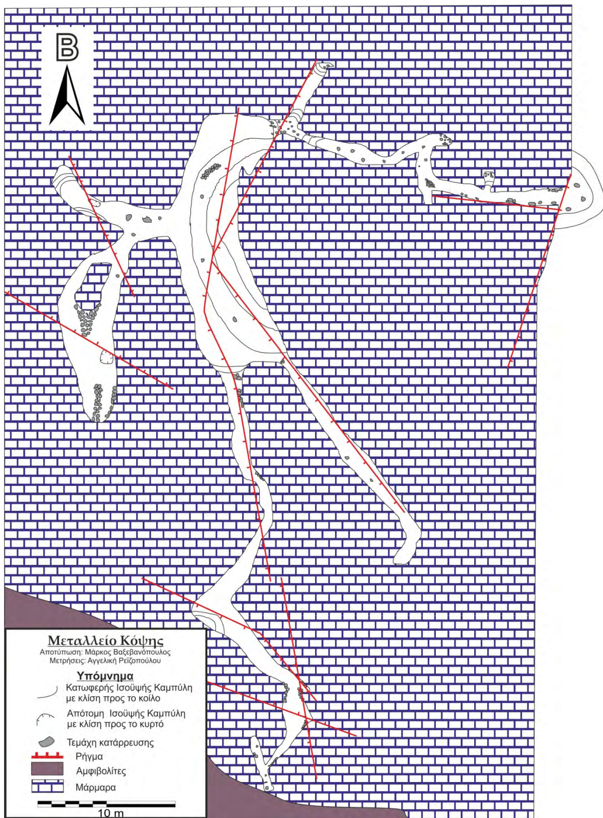
Εικόνα 8.5.3.1 Κάτοψη του μεταλλείου «Κόψης».
