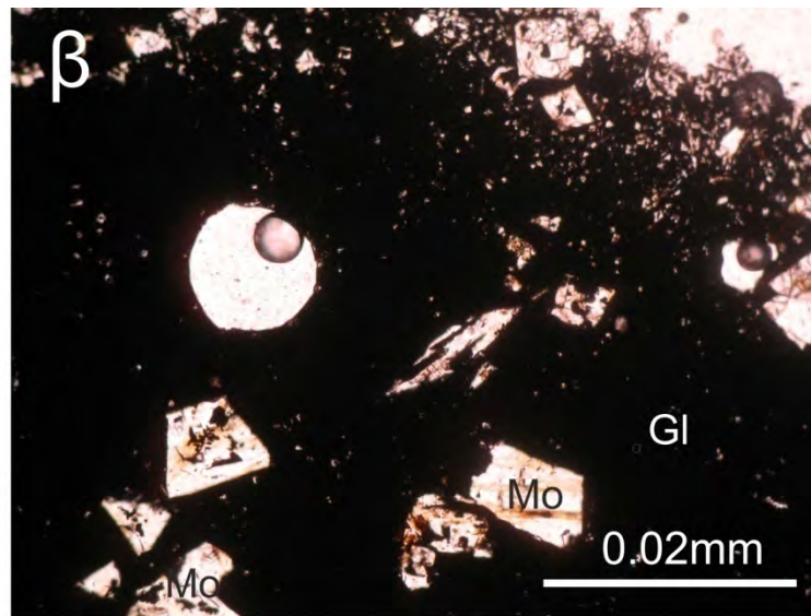
Εικόνα 9.9.2.1 Φωτογραφίες από σκωρίες της περιοχής Ανάληψης. α) Σκωρία με κρυστάλλους βουστίτη (Wus) σε ναλώδη μάζα (Gl) με μοντισελίτη (Mo). Μεταλλογραφικό μικροσκόπιο, //N β) Η φωτογραφία της εικόνας 9.9.4α στο πολωτικό μικροσκόπιο με +N. Διακρίνονται οι κρύσταλλοι του μοντισελίτη (Mo) στην ναλώδη μάζα (Gl). γ) Βουστίτης (Wus) με μοντισελίτη (Mo) σε ναλώδη μάζα (Gl). SEM backscattering image. δ) Κοκκία Pb με βουστίτη (Wus), μοντισελίτη (Mo) σε ναλώδη μάζα (Gl). SEM backscattering image.
