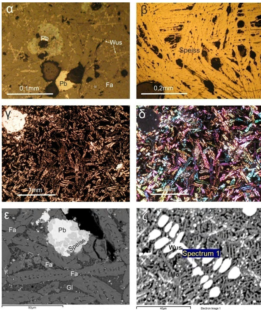
Εικόνα 9.4.2.2 Φωτογραφίες μεταλλουργικών σκωριών από τη Νικήσιανη. α) Δενδριτικές μορφές βουσίτη (Wus) σε φαυαλίτη (Fa) και ναλώδη μάζα (Gl). Διακρίνονται κοκκία Pb. Μεταλλογραφικό μικροσκόπιο, // N. β) Κοκκίο speiss αποτελούμενο από Fe και As. Μεταλλογραφικό μικροσκόπιο, N//. γ) Αλυσιδωτές μορφές κρυστάλλων φαυαλίτη (Fa) μέσα στη μάζα σκωρίας. Πολωτικό Μικροσκόπιο, //N. δ) γ) Αλυσιδωτές μορφές κρυστάλλων φαυαλίτη (Fa) μέσα στη μάζα σκωρίας. Πολωτικό Μικροσκόπιο, +N. ε) Κοκκία μολύβδου (Pb) με speiss μέσα σε μάζα από κρυστάλλους φαυαλίτη (Fa) και ναλώδη μάζα (Gl). SEM back scattering image. ζ) Δενδριτικός βουσίτης (Wus) μέσα σε μάζα από κρυστάλλους μοντισελλίτη (Mo) και ναλώδη μάζα (Gl). SEM back scattering image.
