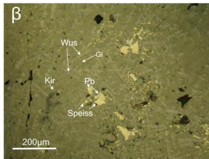
Εικόνα 9.1.2.1 Φωτογραφίες από μεταλλουργικές σκωρίες στο λόφο Σίνα. α) Κοκκίο αποτελούμενο από SPEISS μέσα στη μάζα της μεταλλουργικής σκωρίας. Μεταλλογραφικό μικροσκόπιο //N. β) Δενδριτικός βουστίτης (Wus) με κιρσταϊνίτη (Kir) σε ναλώδη μάζα (Gl). Διακρίνονται τα σφαιρίδια από speiss και μολύβδο (Pb) (λευκοκίτρινο χρώμα). Μεταλλογραφικό μικροσκόπιο //N. γ) Δενδριτικός βουστίτης (Wus), με κιρσταϊνίτη (Kir) μέσα σε ναλώδη μάζα (Gl). Διακρίνονται σφαιρικά κοκκία Speiss με περιεκτικότητες σε Cu από 1 έως 11%. SEM, back scattering image. δ) Κοκκίο Pb και Speiss με περιεκτικότητα σε Cu έως και 18%. Διακρίνεται ο χαλκοσύνης (Cc) με κατάκλαστική υφή. SEM, back scattering image.
