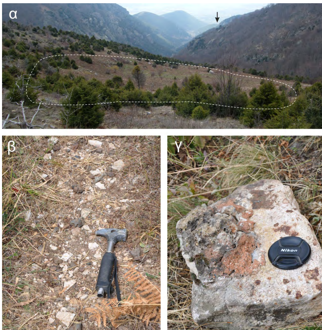
Εικόνα 9.7.1.2 α) Η μεταλλουργική περιοχή Πουλιάνας (στικτή γραμμή) και το χωριό Μεσοροθή στο βάθος (μαύρο βέλος). β) Διάσπαρτες σκωρίες στην περιοχή της Πουλιάνας. γ) Τέμαχος γνευσίου με υπολείμματα αργιλικού υλικού πιθανότατα από τη μεταλλουργική κάμινο.
