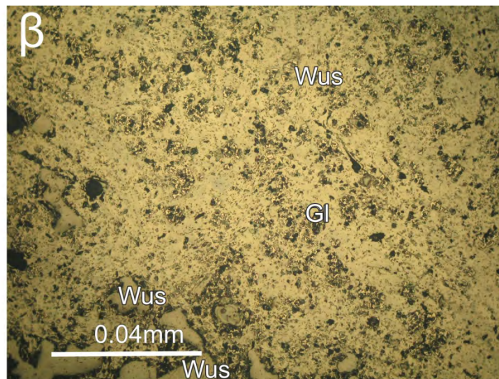
Εικόνα 9.7.2.2 Φωτογραφίες από μεταλλουργικές σκαρίες στην περιοχή Πουλιάνα. α) Κρύσταλλοι κίρσταϊνίτη (Kir) σε ναλώδη μάζα (Gl). Πολωτικό Μικροσκόπιο, //N. β) Η εικόνα 9.7.4β στο μεταλλογραφικό μικροσκόπιο. Διακρίνεται ο βουσιτίτης (Wus), //N. γ) Μεταλλικό κοκκίο Pb-Cu. Διακρίνονται επίσης κρύσταλλοι μοντισελλίτη (Mo), βουσιτίτη (Wus) και η ναλώδης μάζα (Gl). SEM back scattering image. δ) Μεταλλικό κοκκίο Pb-Cu σε κρυστάλλους μοντισελλίτη (Mo) και στην ναλώδη μάζα (Gl) (SEM back scattering image).
