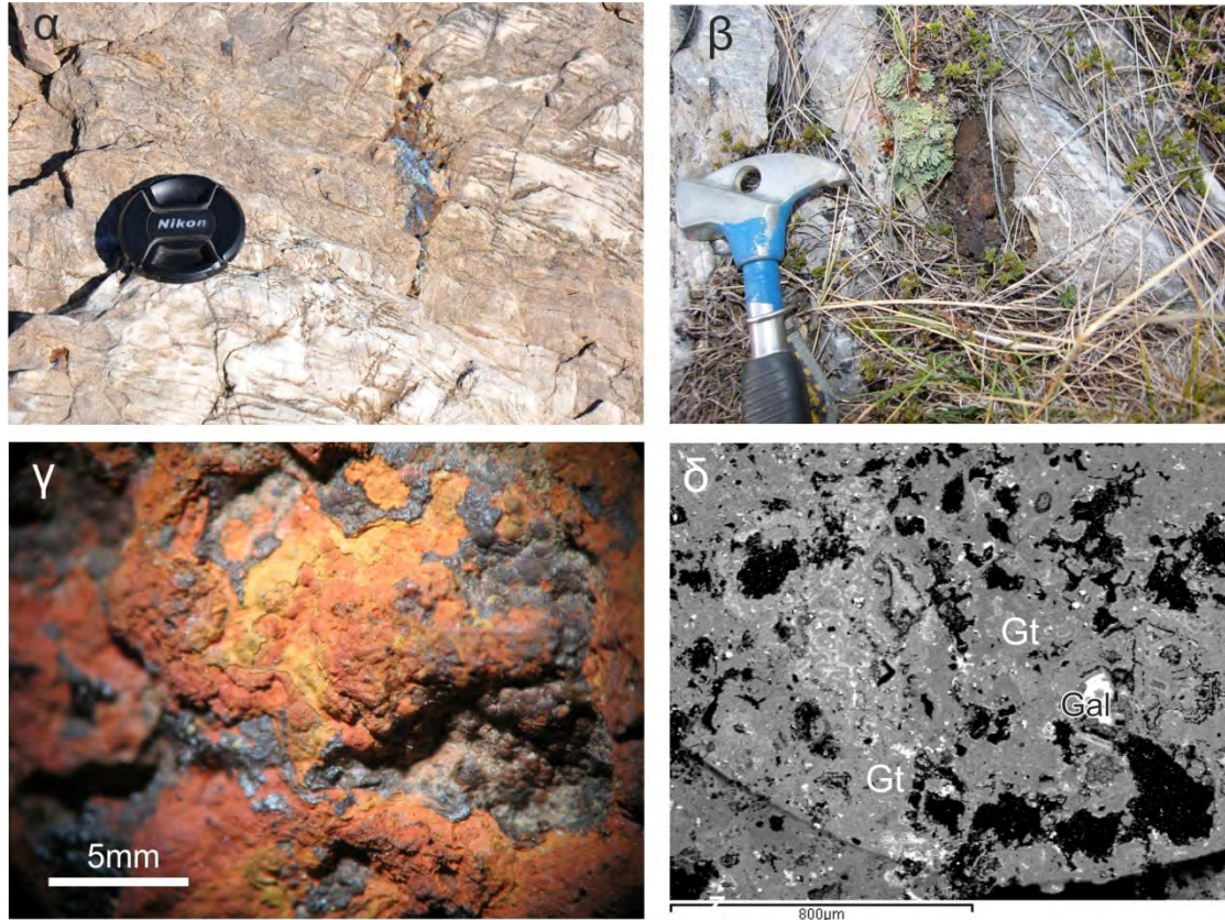
Εικόνα 8.4.5.1 α) Διάκλαση στο μάρμαρο που πληρώνεται από οξειδωμένη μεταλλοφορία γκαιτίτη, μαλαχίτη, αζουρίτη στην περιοχή Αβγού. β) Διάκλαση πληρωμένη με γκαιτίτη-σιδηροπυρίτη. γ) Μεταλλοφορία με γκαιτίτη από τις εκβολάδες της μεταλλευτικής στοάς Αβγό-1. δ) Γκαιτίτης (Gt) και γαληνίτης (Gal) από τη μεταλλοφορία του Αβγού. SEM, back scattering image.
