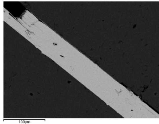
Εικόνα 8.7.5.2 Επιμήκης κρύσταλλος τσουμοϊτη πλούσιου σε Pt (ορυκτό Β) μέσα σε σιδηροπυρίτη από την περιοχή της Νεροστριάς. SEM, back-scattering image.
