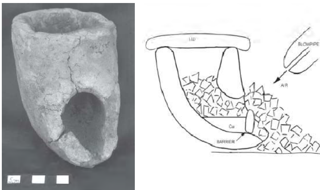
Εικόνα 3.8.2.3 Αιγυπτιακό χωνευτήριο και τομή κατά τη διαδικασία εκκαμίνευσης (Davey and Edwards, 2007).
