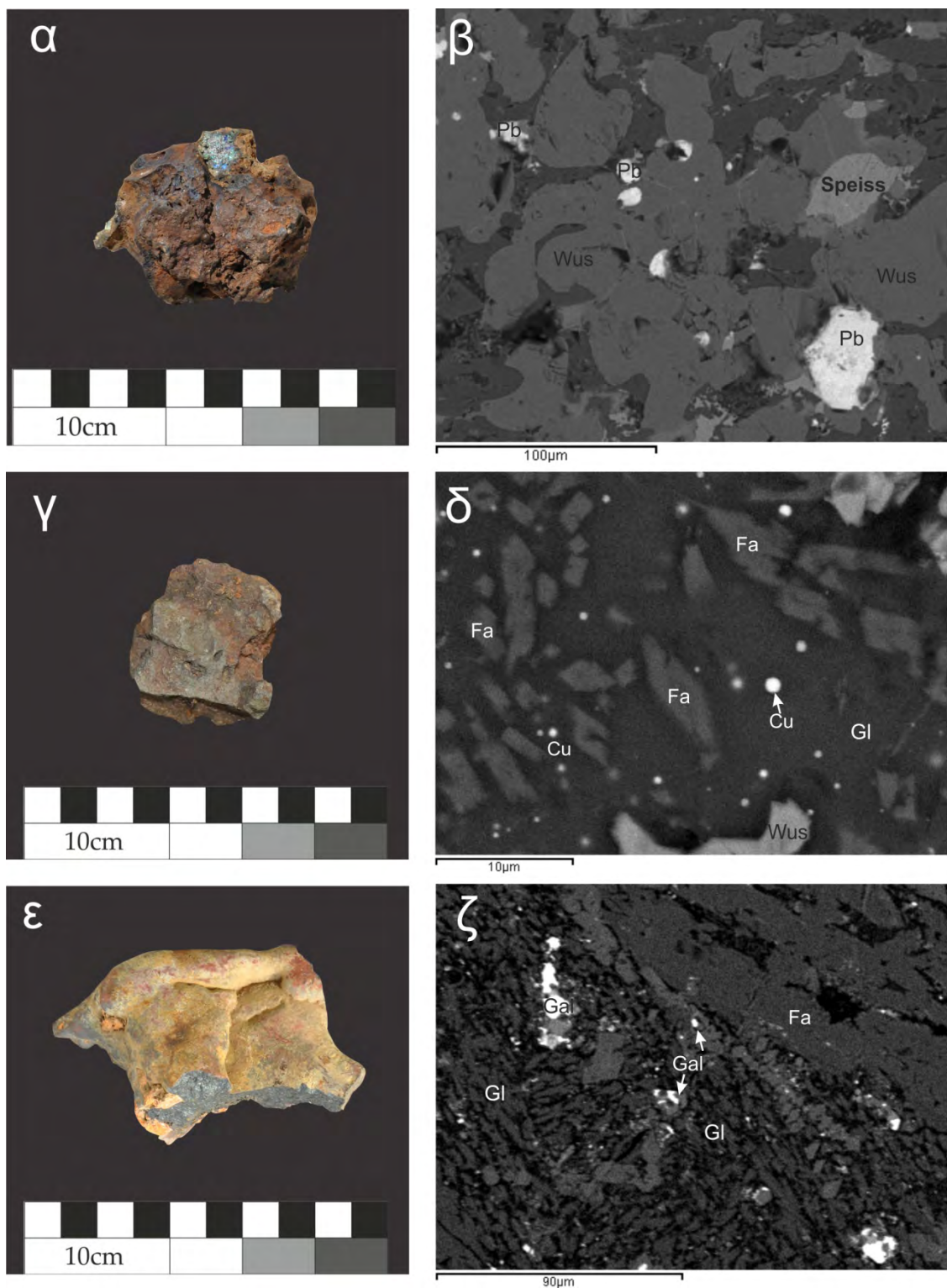
Εικόνα 9.5.2.2 α) Σκωρία Α' ομάδας β) Σκωρία Α' ομάδας όπου διακρίνονται κοκκία Pb και speiss σε μάζα από βουστίτη (Wu) και ναλώδη μάζα (Gl). SEM back scattering image. γ) Σκωρία Β' ομάδας δ) Σκωρία Β' ομάδας με κοκκία χαλκού (Cu) και κρυστάλλους φαυαλίτη (Fa) σε ναλώδη μάζα (Gl). SEM back scattering image. ε) Σκωρία Γ' ομάδας ζ) Σκωρία Γ' ομάδας με γαληνίτη (Gal) μέσα σε μάζα από φαυαλίτη (Fa) και ύαλο (Gl). SEM back scattering image.
