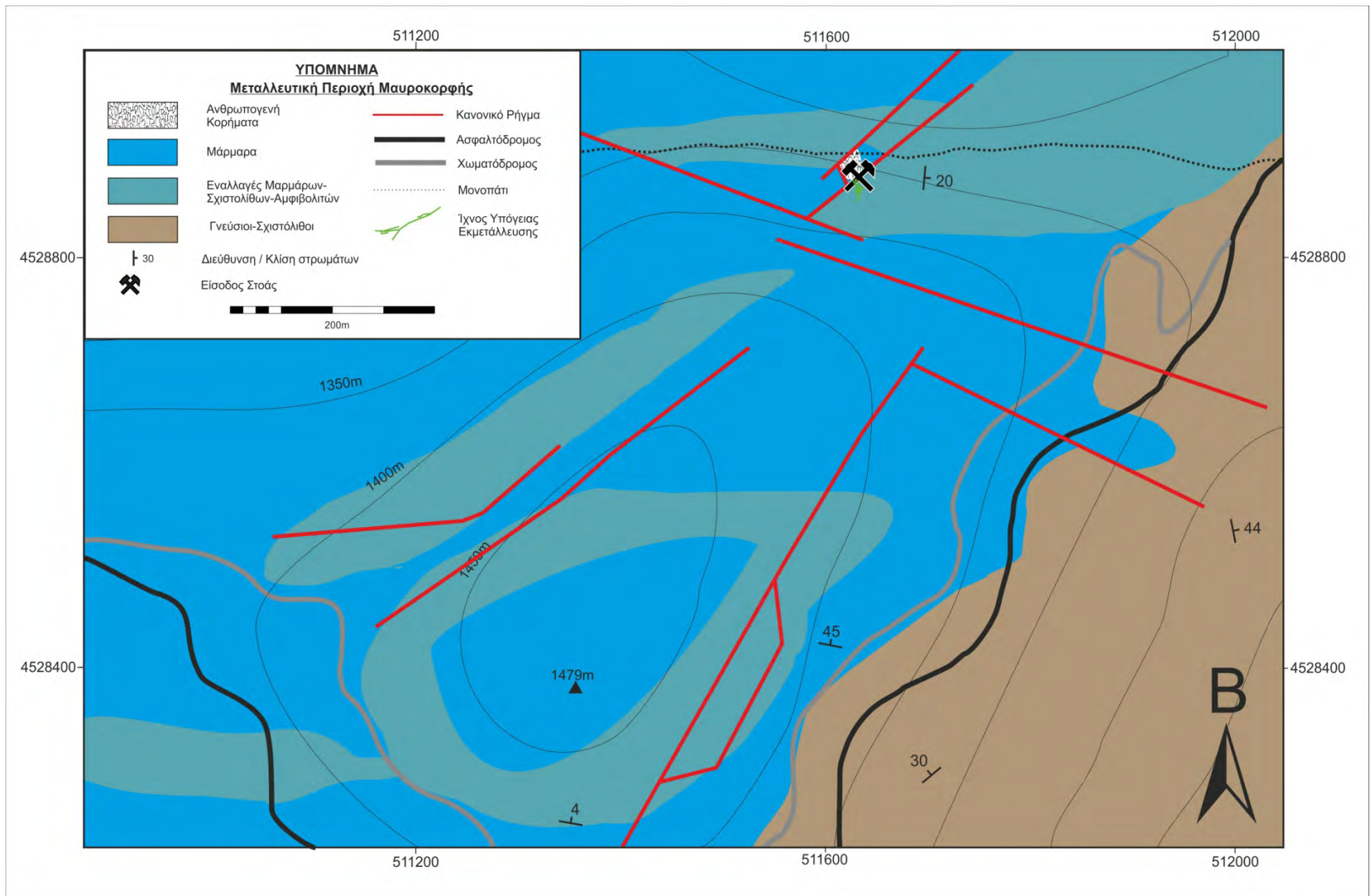
Εικόνα 8.3.2.2 Γεωλογικός χάρτης (κάτοψη) της μεταλλευτικής περιοχής Μαυροκορφής.
