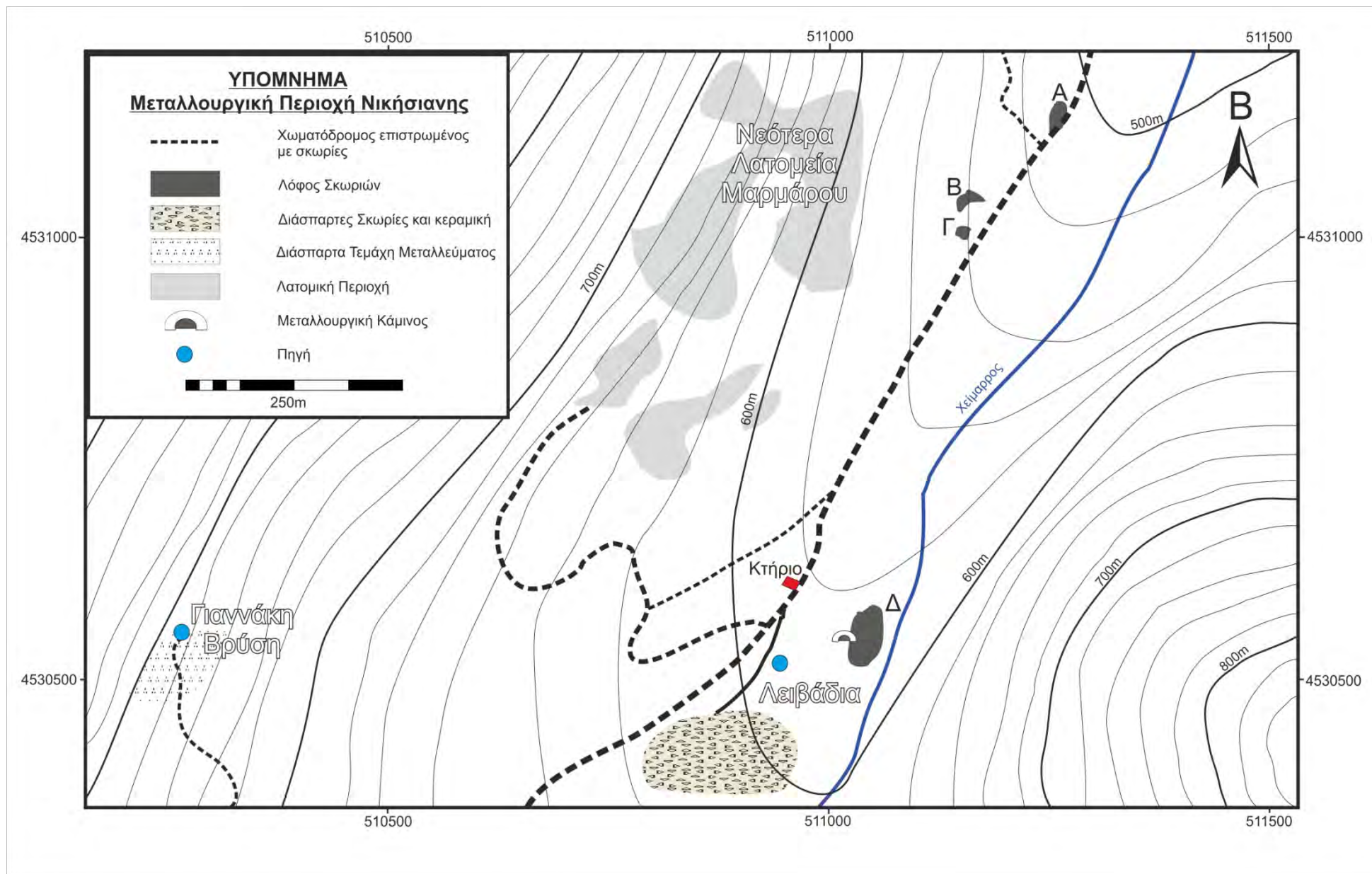
Εικόνα 9.4.1.2 Χάρτης της μεταλλουργικής περιοχής Νικήσιανης.
