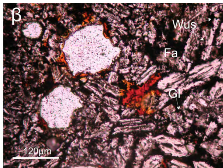
Εικόνα 9.3.2.2 Φωτογραφίες σε μικροσκόπιο από σκωρίες στη μεταλλουργική θέση Παλαιοχωρίου α) Βουσιτίτης (Wus) σε φαυαλίτη (Fa). Οι βαθύχρωμες φάσεις είναι η υαλώδης μάζα (Gl), ενώ διακρίνονται οι σπές της σκωρίας. Μεταλλογραφικό μικροσκόπιο, N//. β) Η φωτογραφία 9.3.5α με πολωτικό μικροσκόπιο. Διακρίνονται οι επιμήκεις κρύσταλλοι του φαυαλίτη. N//. γ) Φαυαλίτης (Fa) μέσα σε υαλώδη μάζα (Gl). Με λευκό χρώμα διακρίνεται ο βουσιτίτης (Wus). SEM Back scattering image. δ) Επιμήκεις κρύσταλλοι φαυαλίτη (Fa) μέσα σε υαλώδη μάζα (Gl). Με λευκό χρώμα διακρίνεται ο βουσιτίτης (Wus). SEM Back scattering image.
