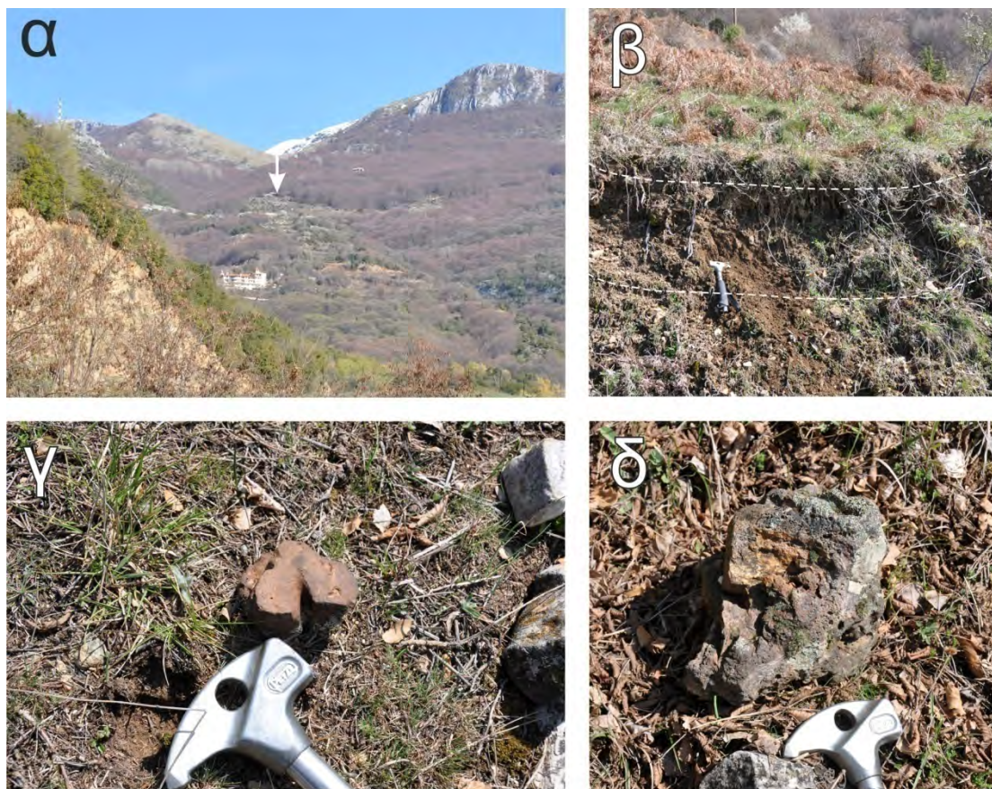
Εικόνα 9.9.1.2 α) Μεταλλουργική περιοχή Ανάληψης (βέλος) πάνω από τη Μονή Αναλήψης. β) Στρώμα με διάσπαρτες μεταλλουργικές σκωρίες. γ) Συμπαγής επιφανειακή σκωρία στη θέση Ανάληψη. δ) Τμήμα γνευσίου με αργιλικό συνδετικό υλικό από τοίχωμα μεταλλουργικής καμίνου.
