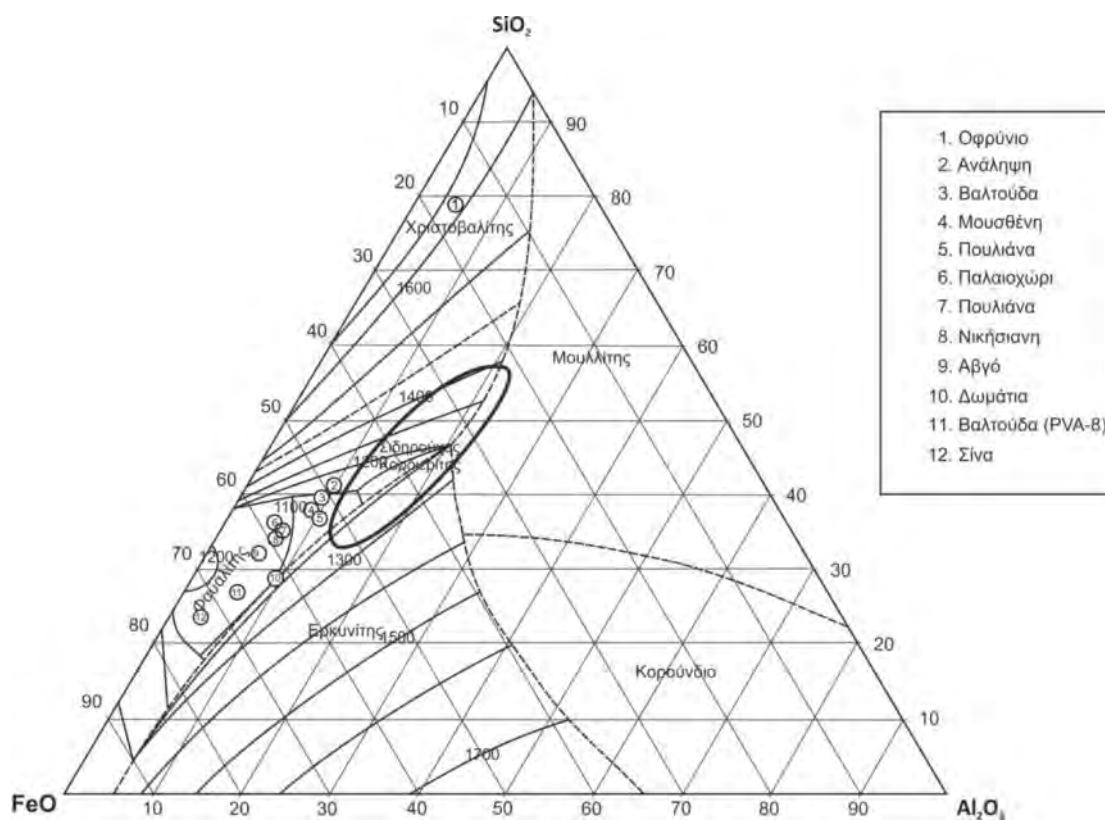
Εικόνα 11.3.4 Τριγωνικό διάγραμμα ( \text{SiO}_2\text{-FeO-Al}_2\text{O}_3 ) των δειγμάτων σκωριών από το όρος Παγγαίο.
