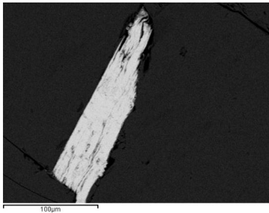
Εικόνα 8.7.5.1 Επιμήκης κρύσταλλος τσουμοϊτη πλούσιου σε Pb (ορυκτό Α) μέσα σε σιδηροπυρίτη από την περιοχή της Νεροστριάς. SEM, back-scattering image.
