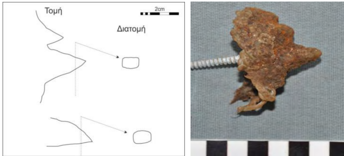
Εικόνα 8.5.3.4 Σχηματική απεικόνιση των ιχνών εκμετάλλευσης (αριστερά) με βάση θετικά εκμαγεία του μεταλλευτικού σφυριού (δεξιά) από το εσωτερικό του μεταλλείου Κόψης.
