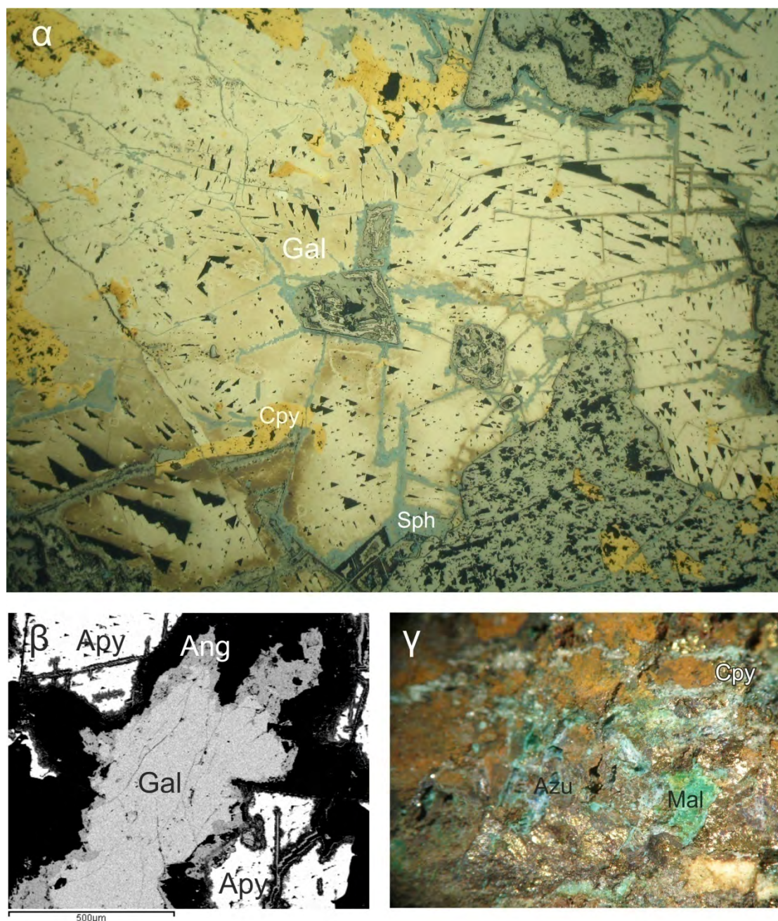
Εικόνα 8.6.10.3 α) Γαληνίτης (Gal), χαλκοπυρίτης (Cpy) και σφαλερίτης (Sph) από την πρωτογενή μεταλλοφορία στις Ασημότρυπες. //N Μήκος φωτογραφίας 500 μm (Μεταλλογραφικό μικροσκόπιο) β) Γαληνίτης (Gal) περιτοιχισμένος από κρυστάλλους αρσеноπυρίτη (Apy). Στα όριά του μεταπίπτει σε αγγλεσίτη (Ang). Εικόνα από ηλεκτρονικό μικροσκόπιο. γ) Χαλκοπυρίτης (Cpy) που έχει μετατραπεί σε μαλαχίτη (Mal) και αζουρίτη (Azu). Μήκος φωτογραφίας 0,8 mm (Εικόνα από στερεοσκόπιο).
