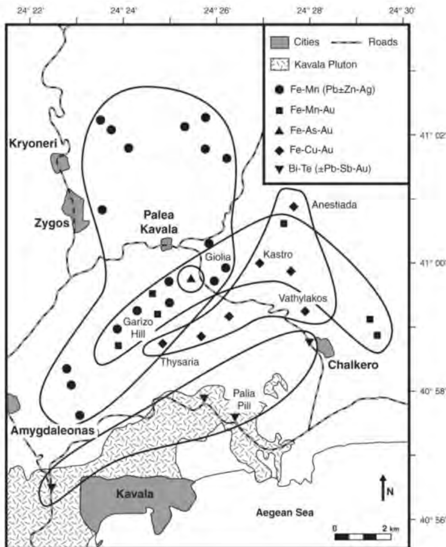
Εικόνα 5.6.2 Ζώνες μεταλλοφορίας στην περιοχή της Παλαιάς Καβάλας. Η μεταλλοφορία Bi-Te ( \pm Pb-Sb-Au) εντοπίζεται πλησίον του πλουτωνίτη της Καβάλας (Fornadel et al, 2011 τροποποιημένο από Vavelidis et al, 1997b).
