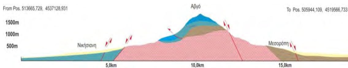
Εικόνα 7.1.2 Γεωλογική τομή του όρους Παγγαίου διεύθυνσης ΒΑ-ΝΔ. Η υπομνημάτιση των γεωλογικών σχηματισμών στο γεωλογικό χάρτη της προηγούμενης σελίδας. (Τροποπ. από Kronberg, 1972; Kronberg and Schenck, 1974; Ξυδά, 1978 και παρατηρήσεις κατά το παρόν πόνημα).
