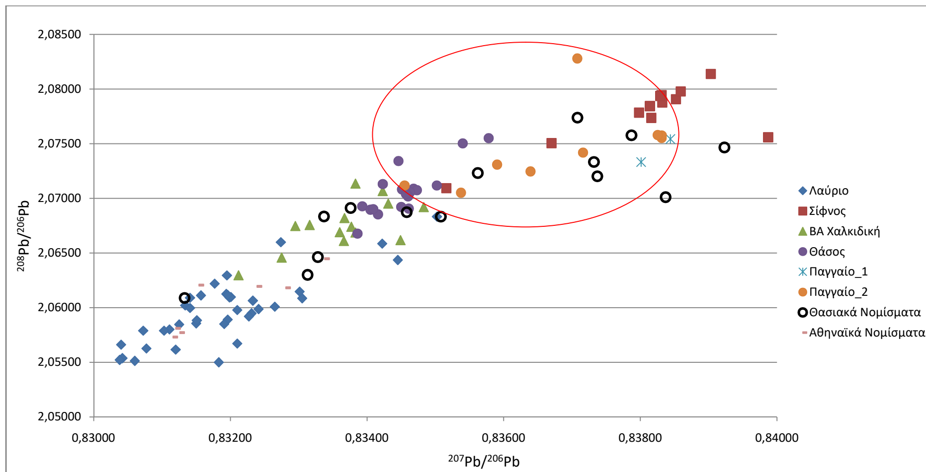
Σχήμα 10.2.6 Ισοτοπικές αναλογίες ( ^{207}\text{Pb}/^{206}\text{Pb} προς ^{208}\text{Pb}/^{206}\text{Pb} ) δειγμάτων από μετάλλευμα και σκωρίες από το Λαύριο, τη Σίφνο, τη ΒΑ Χαλκιδική, τη Θάσο και το Παγγαίο. Επιπλέον τοποθετούνται και ισοτοπικά δεδομένα από αρχαία νομίσματα από τη νήσο Θάσο και από την Αττική. Οι αναλύσεις των δειγμάτων προέρχονται από τη βάση δεδομένων OXALID (Gale et al, 1980; 1988) εκτός της ομάδας Παγγαίο_2 που προέρχονται από την παρούσα έρευνα. Σημειώνεται το πεδίο ισοτόπων του όρους Παγγαίου, όπου περικλείονται αρκετά νομίσματα από τη νήσο Θάσο.
