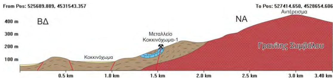
Εικόνα 8.1.2.1 Γεωλογική τομή στην περιοχή του Κοκκινόχωματος (τροποποιημένο από Kronberg and Schenck, 1974, υπόμνημα όπως στην Εικ. 7.1.1).
