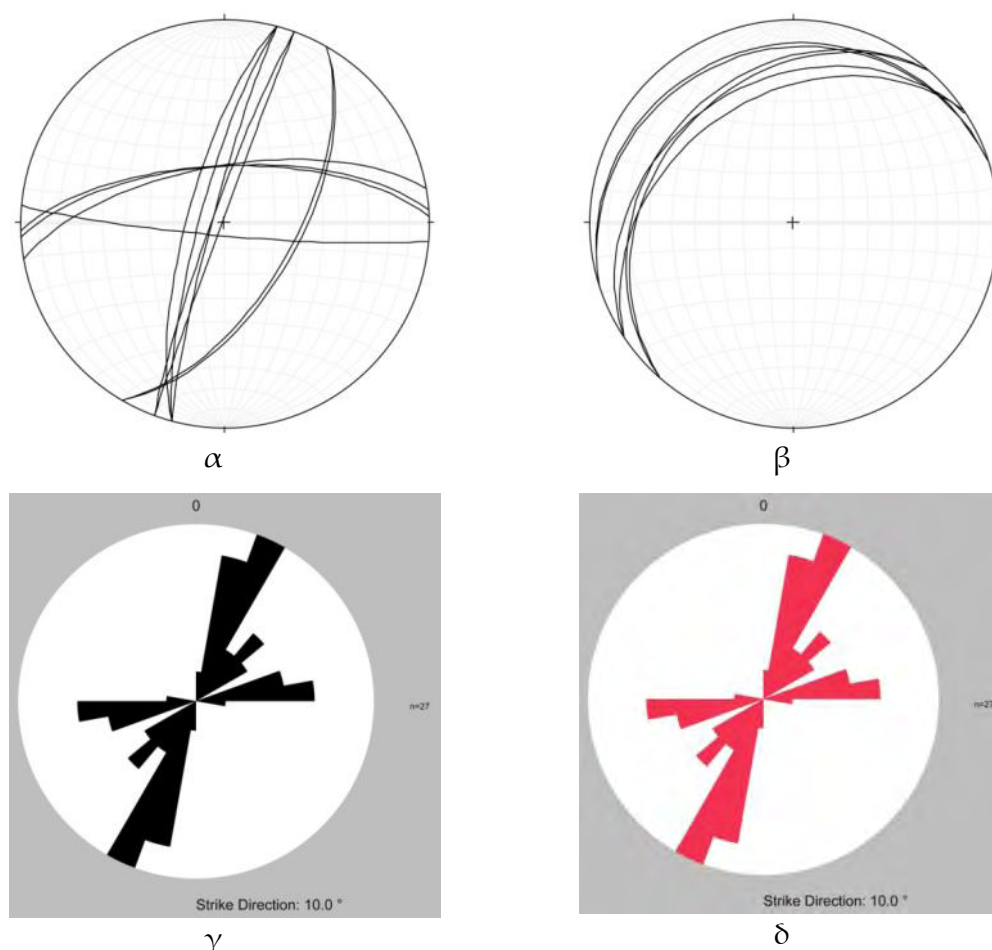
Σχήμα 8.1.2.1 Στερεογραφικές προβολές (κάτω ημισφαίριο) και ροδοδιαγράμματα των ασυνεχειών από το εσωτερικό της στοάς «Κοκκινόχωμα-1». α. Προβολή των τεκτονικών ασυνεχειών και των μέγιστων πόλων. β. Προβολή των επιφανειών σχιστότητας. γ. Ροδοδιάγραμμα των ασυνεχειών της στοάς. δ. Ροδοδιάγραμμα ασυνεχειών που φιλοξενούν μεταλλοφορία.
