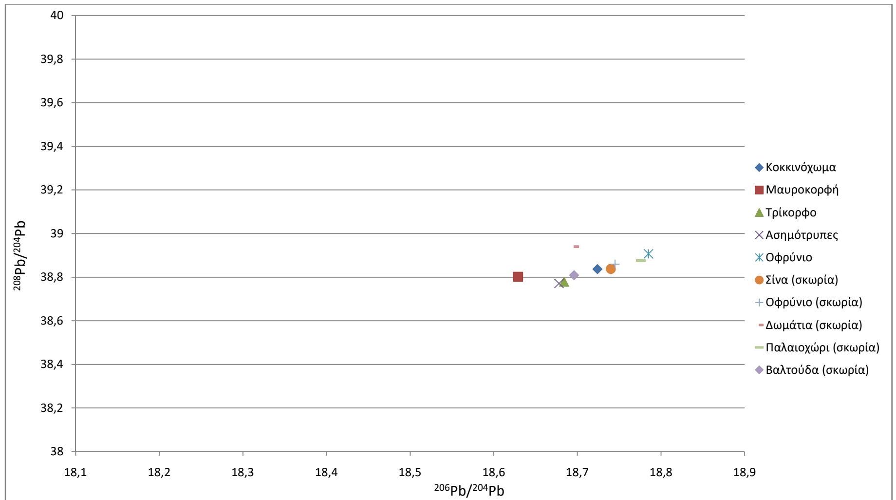
Σχήμα 10.9.3 Ισοτοπικές αναλογίες ( ^{206}\text{Pb}/^{204}\text{Pb} προς ^{208}\text{Pb}/^{204}\text{Pb} ) δειγμάτων από μεταλλεία και μεταλλουργικές περιοχές από την ευρύτερη περιοχή του Παγγαίου όρους. Παρατηρείται σχετικά γραμμική ανάπτυξη πλην του δείγματος από τη μεταλλουργική θέση των «Δωματίων».
