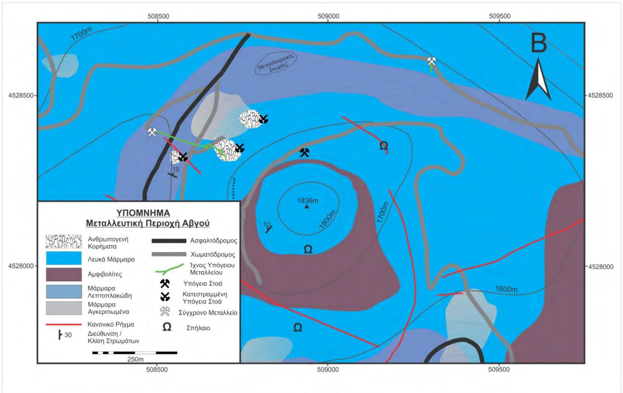
Εικόνα 8.4.2.2 Γεωλογικός χάρτης (κάτοψη) μεταλλευτικής περιοχής Αβγού.
