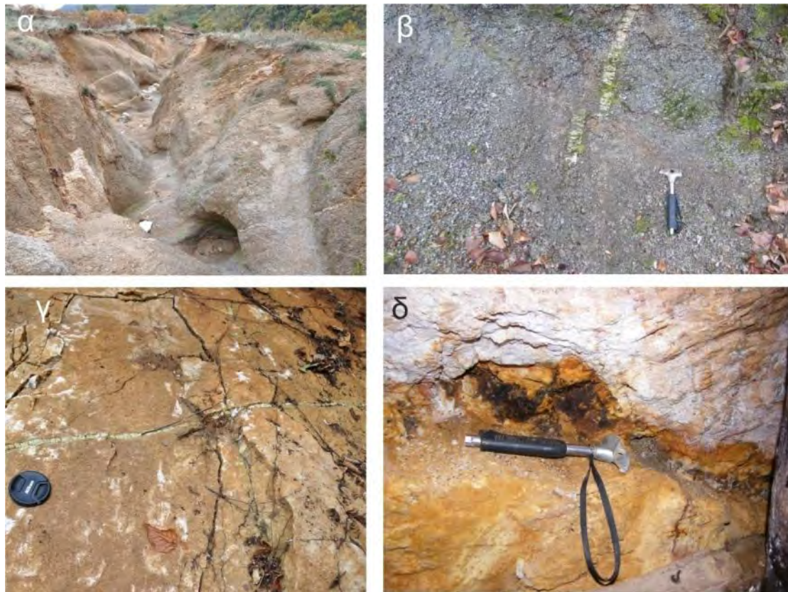
Εικόνα 8.7.2.1 α) Ο γρανίτης όπως αποκαλύπτεται σε σημεία έντονης διάβρωσης. β) Μετατοπισμένη πηγματιτική φλέβα από ρήγμα. γ) Φλέβα δευτερογενούς ασβεσίτη στη μάζα των μαρμάρων. δ) Φωλιά μεταλλεύματος στην επαφή του πλουτωνίτη με τα υπερκείμενα μάρμαρα της περιοχής.
