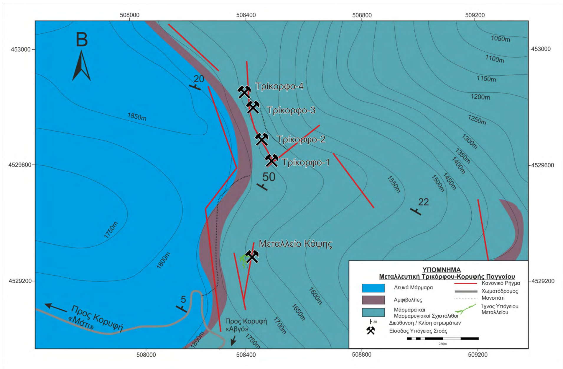
Εικόνα 8.5.2.4 Γεωλογικός χάρτης (κάτοψη) μεταλλευτικής περιοχής Τρίκορφου-Κορυφής Παγγαίου.
