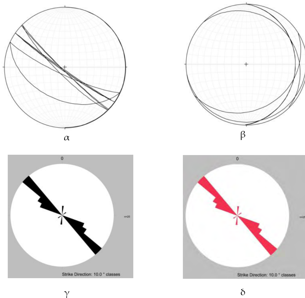
Σχήμα 8.7.2.1 Στερεογραφικές προβολές (κάτω ημισφαίριο) και ροδοδιαγράμματα των ασυνεχειών από το εσωτερικό της στοάς «Νεροστριά-1». α. Προβολή των τεκτονικών ασυνεχειών. β. Προβολή των επιφανειών σχιστότητας. γ. Ροδοδιάγραμμα των τεκτονικών ασυνεχειών της στοάς. δ. Ροδοδιάγραμμα τεκτονικών ασυνεχειών που φιλοξενούν μεταλλοφορία.
