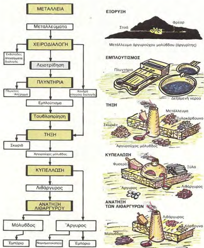
Εικόνα 3.8.5.1 Η αλυσίδα παραγωγής αργύρου και μολύβδου στο αρχαίο Λαύριο (Κονοφάγος, 1980).
