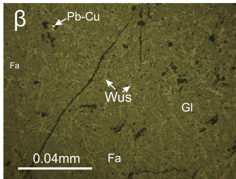
Εικόνα 9.8.2.1 Φωτογραφίες μεταλλουργικών σκωριών από τη θέση Αβγόα) Συμπαγής σκωρία από τη μεταλλουργική θέση του Αβγού β) Κρύσταλλοι βουσίτη (Wus) σε φαυαλίτη (Fa) και υαλώδη μάζα (Gl) Επίσης διακρίνονται μεταλλικά κοκκία Pb-Cu. Μεταλλογραφικό μικροσκόπιο //N. γ) Κοκκίο Pb-Cu σε βουσίτη (Wus) και φαυαλίτη (Fa). Επίσης διακρίνεται στη μάζα της σκωρίας γαληνίτης (Gal). Υαλώδης μάζα (Gl). SEM back scattering image. δ) Κοκκίο Pb-Cu. SEM back scattering image.
