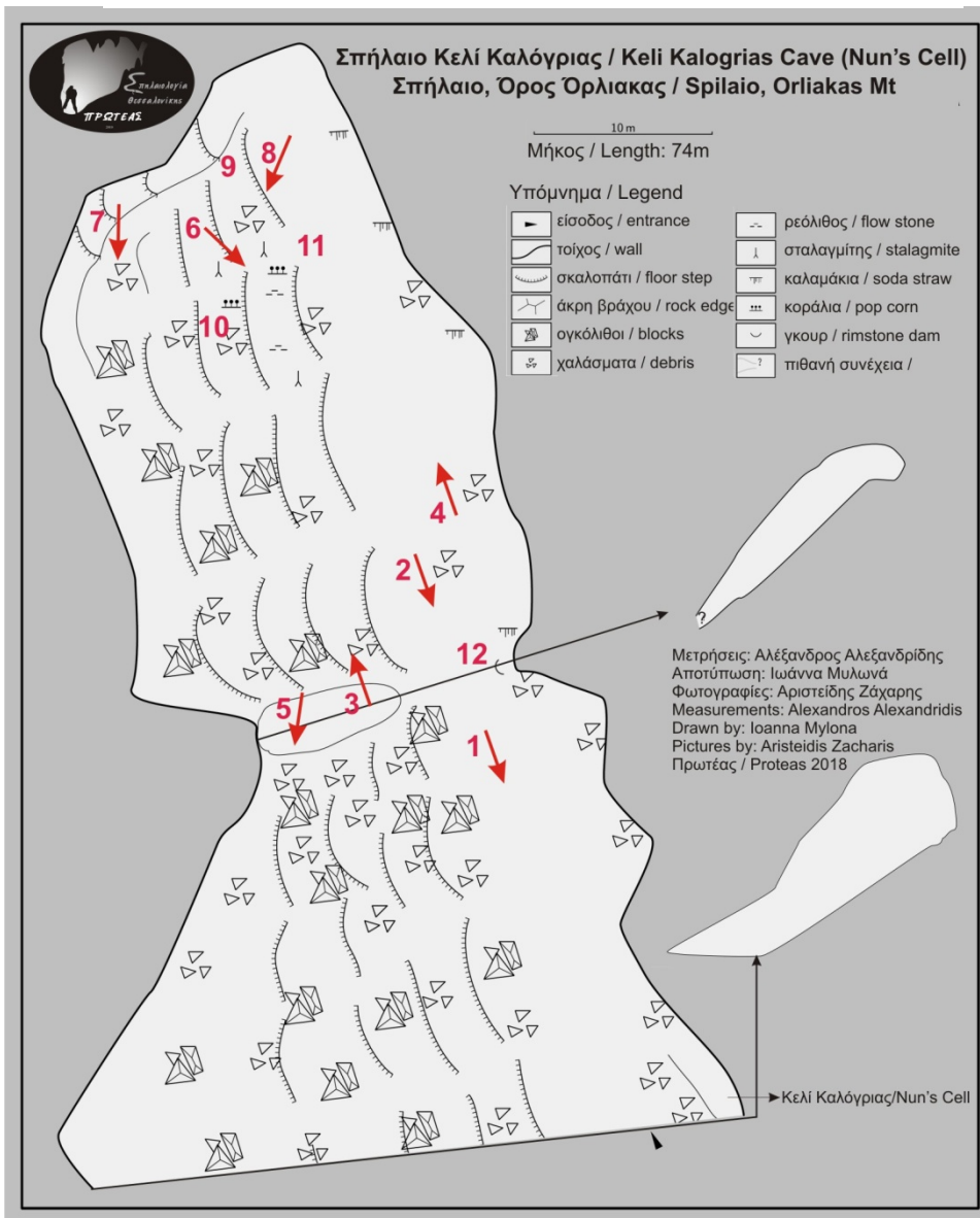
Εικόνα 14 – Χαρτογράφηση Κελί Καλόγριας
