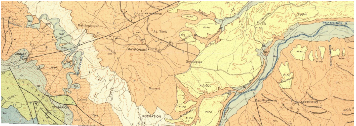
Γεωλογικός χάρτης της περιοχής. Με πράσινο ο ασβεστολιθικός όγκος του Όρλιακα
